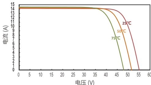
JT610SRt(B) 不同温度下的IV曲线
