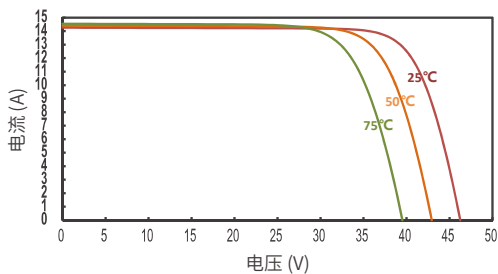
JT475Slt(B) 不同温度下的IV曲线
