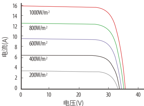
JT445Snt(B) 不同光强下的PV曲线
