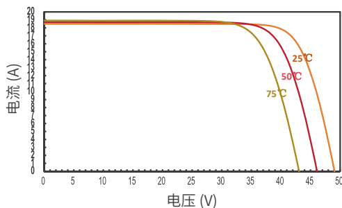
JT715SPt(B) 不同温度下的IV曲线
