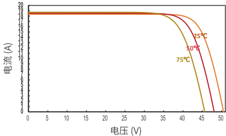
JT730SLk(B) 不同温度下的IV曲线
