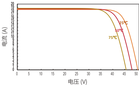
JT730SLk(B) 不同温度下的IV曲线
