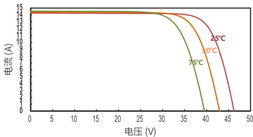
JT515SLt(B) 不同温度下的IV曲线
