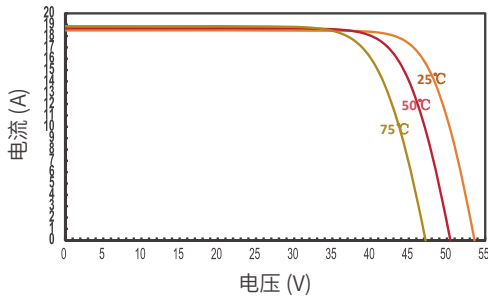
JT780SXt(B) 不同温度下的IV曲线
