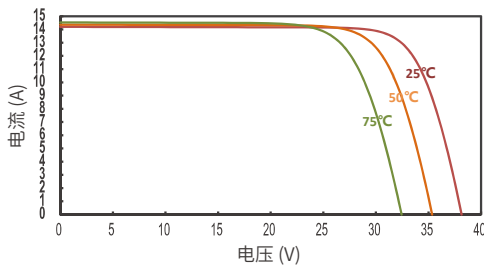
JT425Sjt(B) 不同温度下的IV曲线
