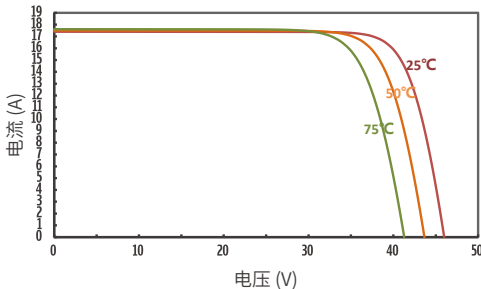
JT640SIk(B) 不同温度下的IV曲线
